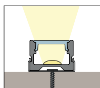
Montering med clips
